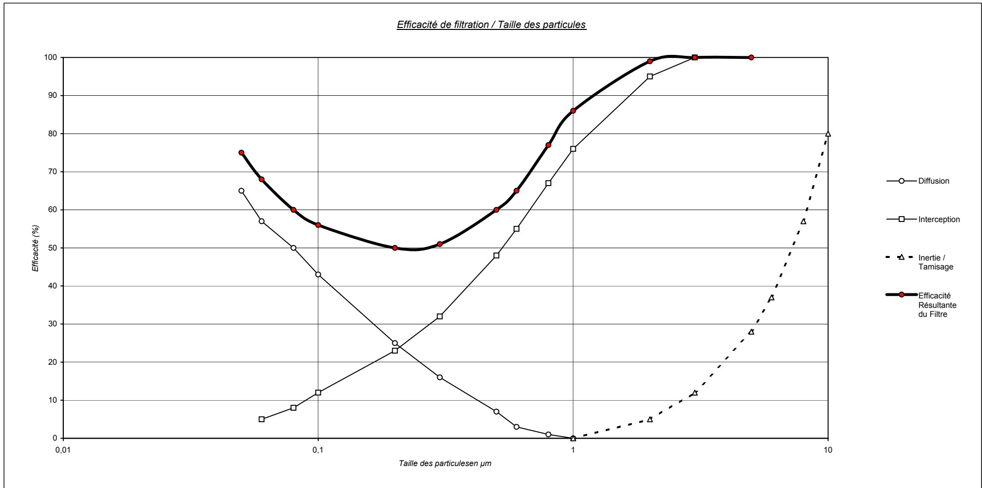
TAMISAGE
